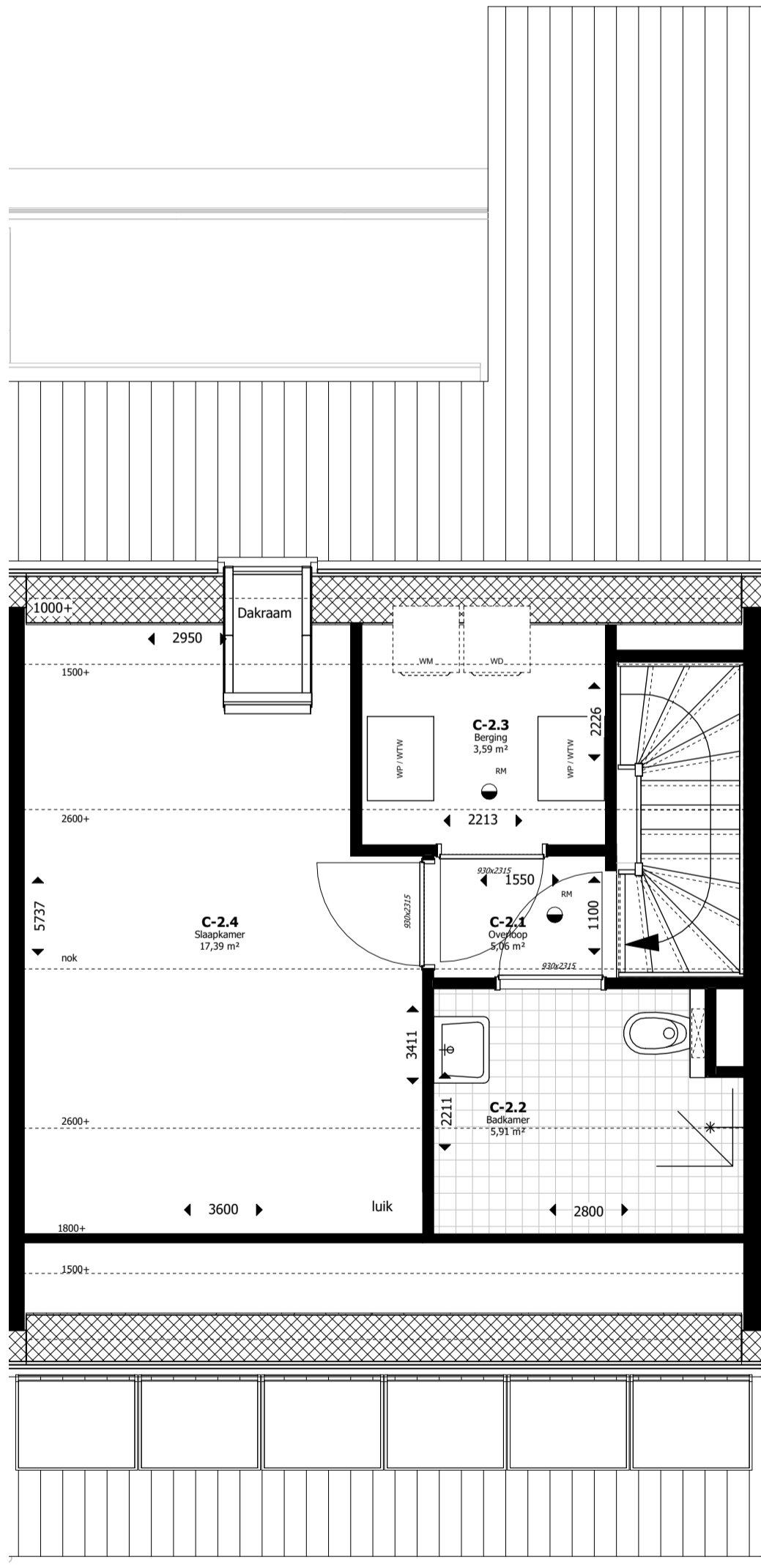
Verdieping 2
