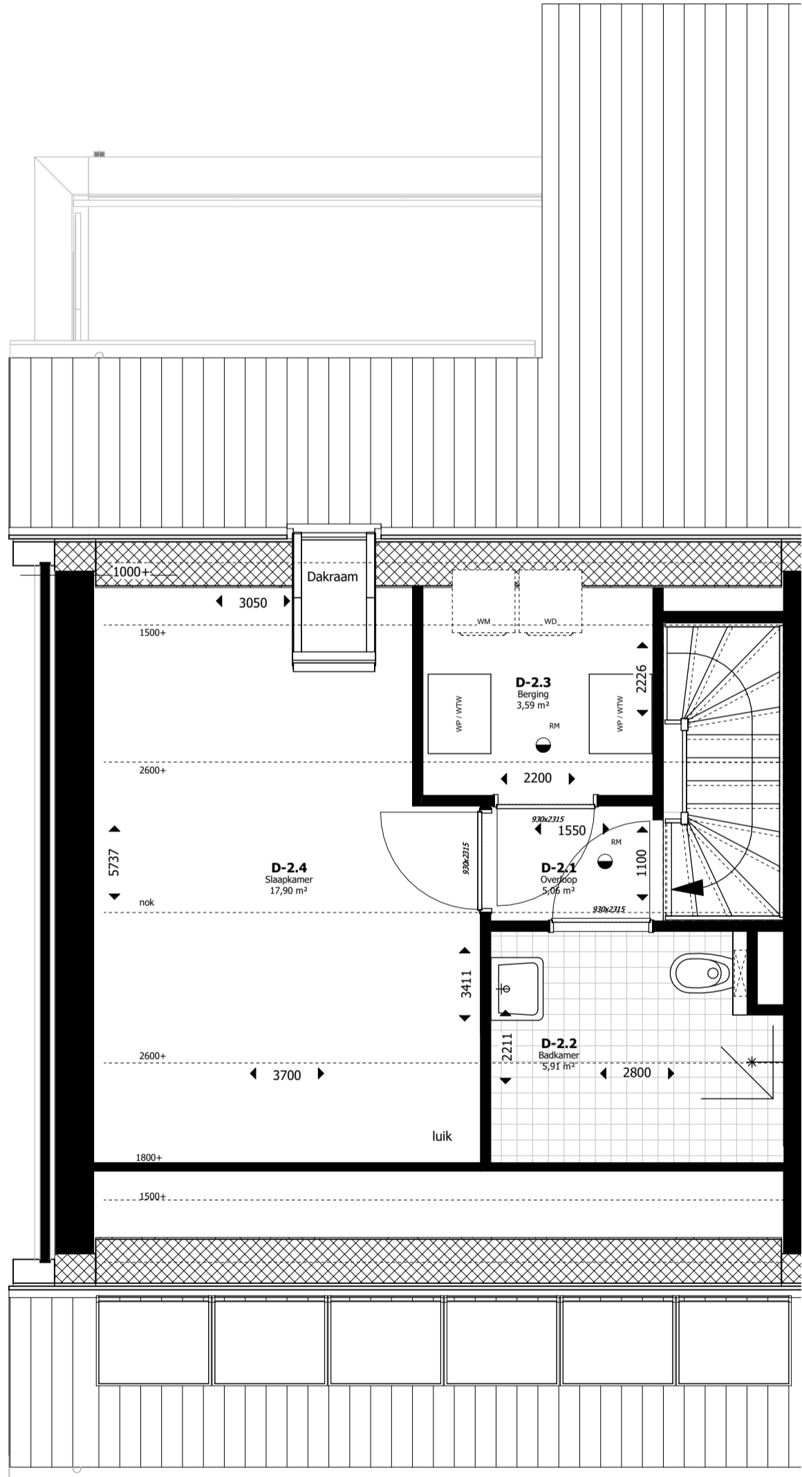
Verdieping 2
