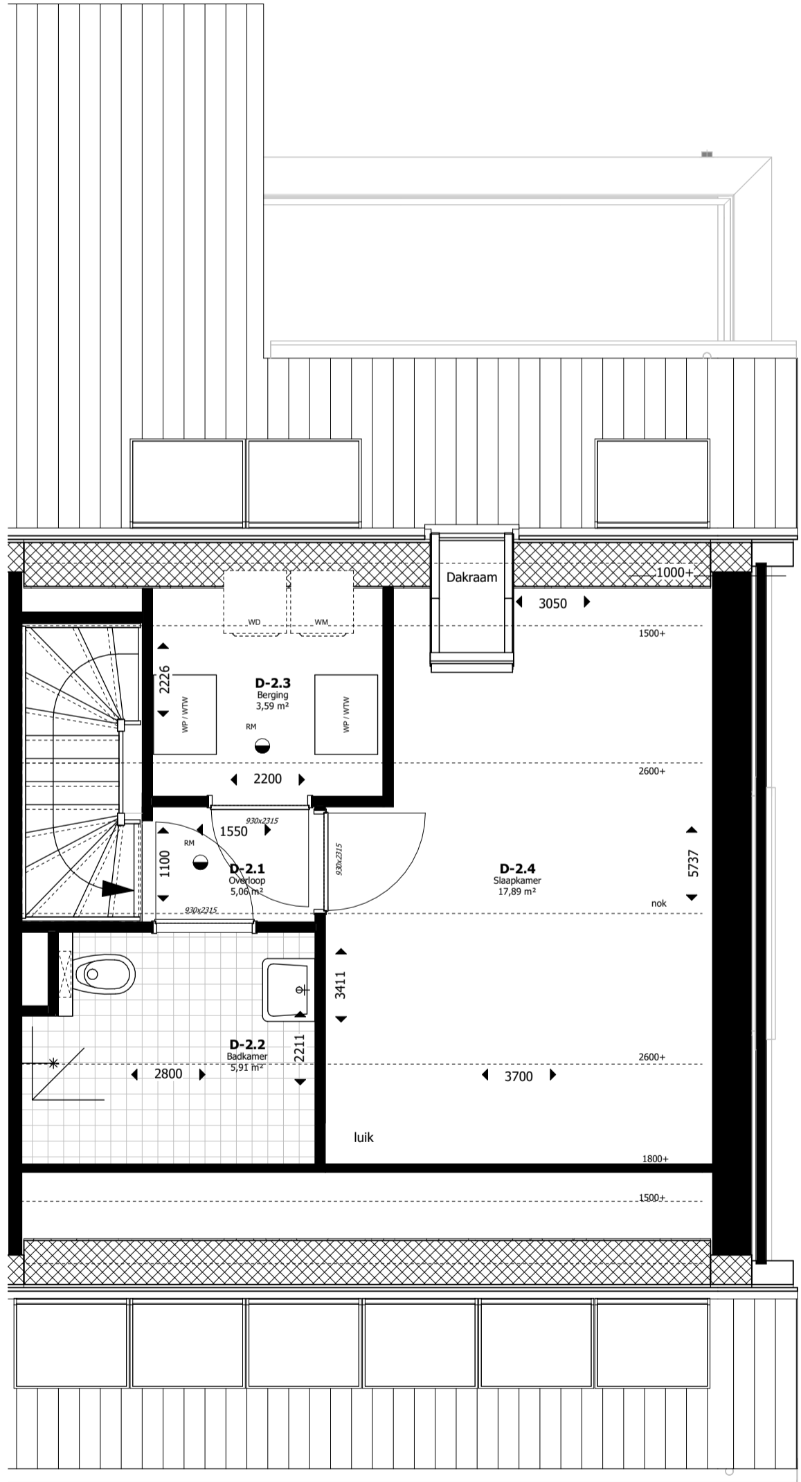
Verdieping 2
