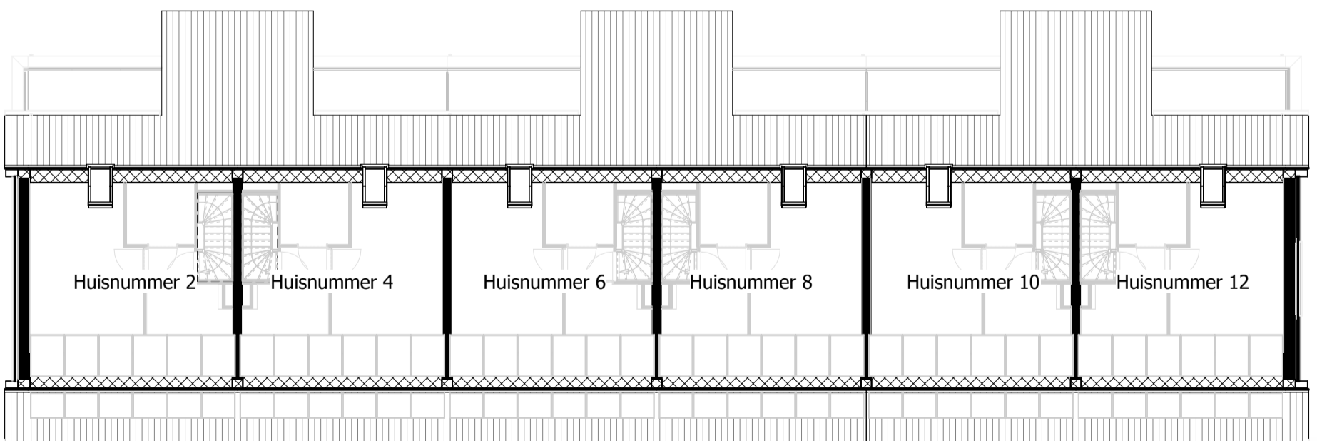
Verdieping 2
