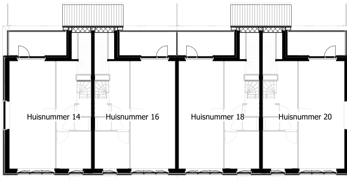
Verdieping 1
