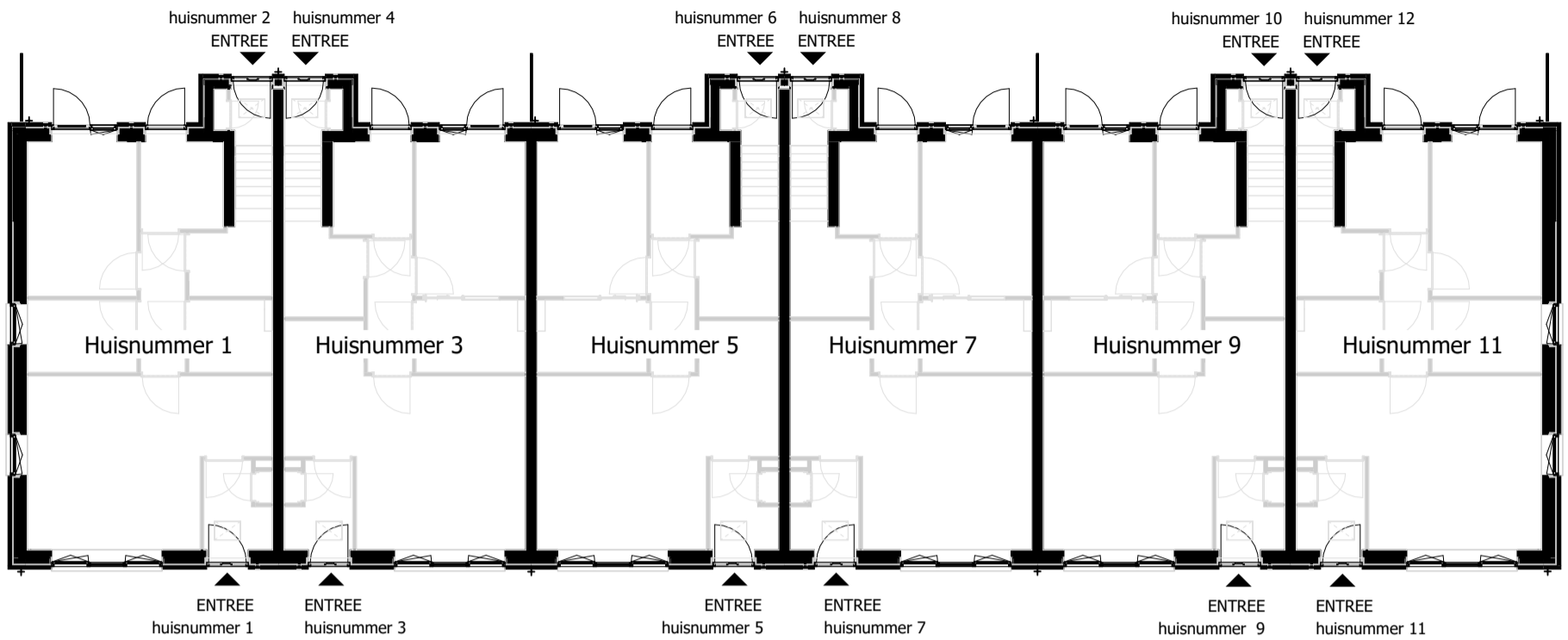
Begane grond
