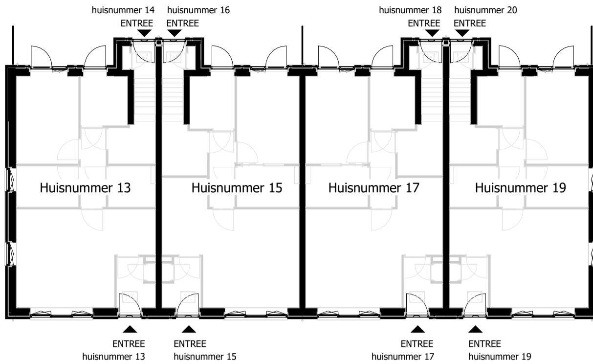
Begane grond
